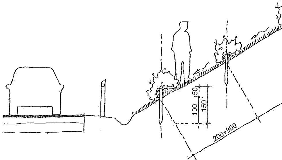
□ Sezione
