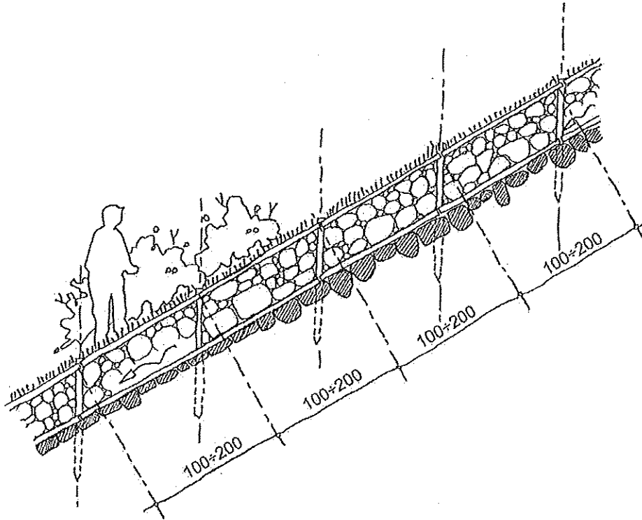
□ Profilo longitudinale
