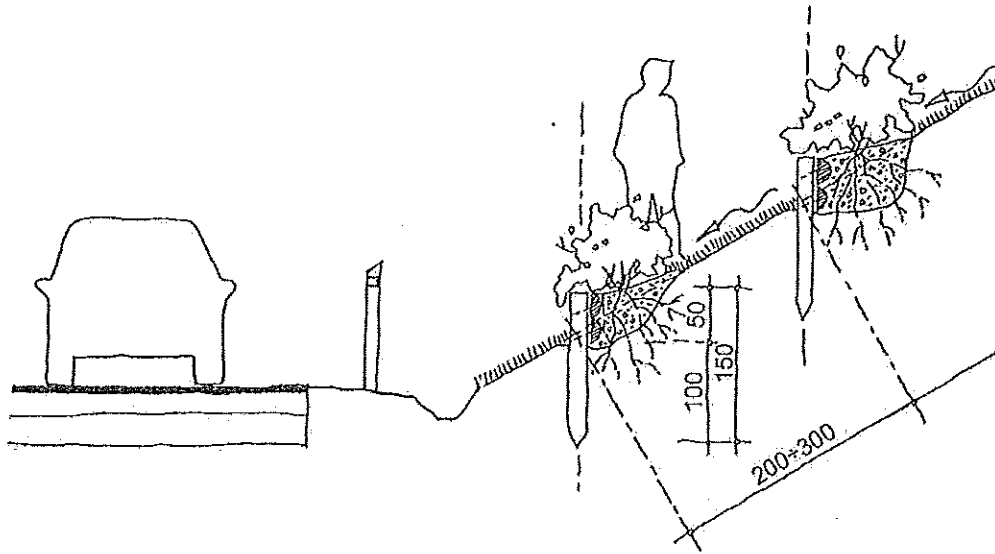
Sezione
